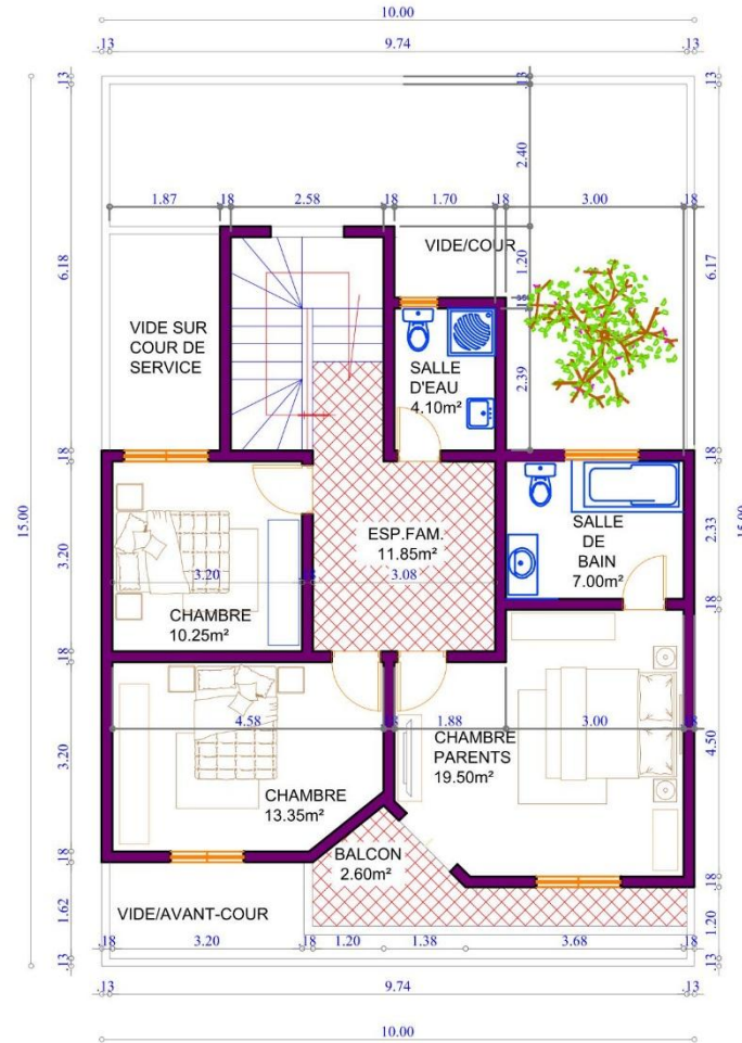
PLAN ETAGE
