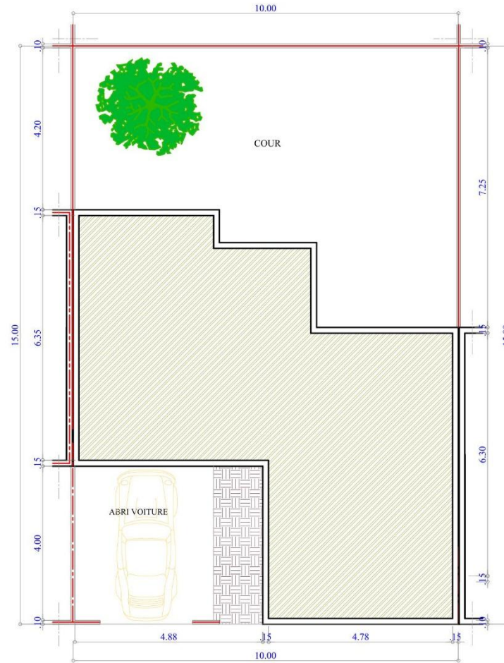
PLAN TOITURE
