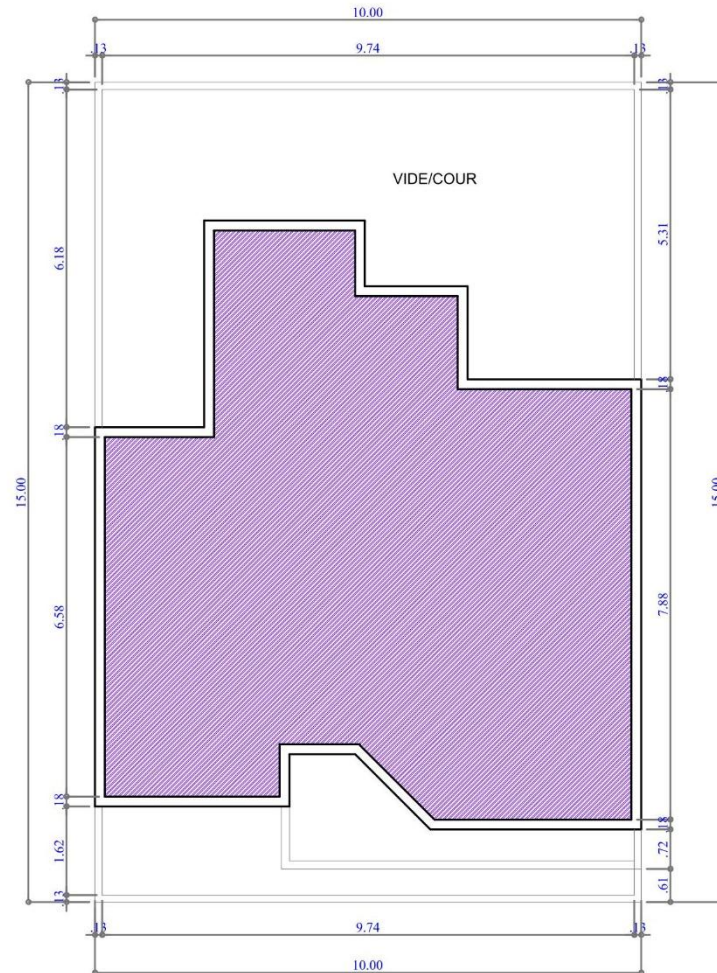
PLAN DE TOITURE
