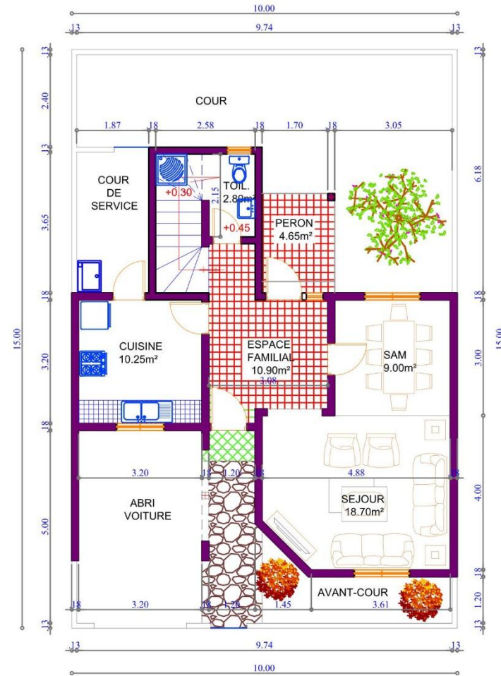
PLAN REZ-DE-CHAUSSEE
