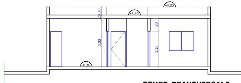
COUPE TRANSVERSALE
