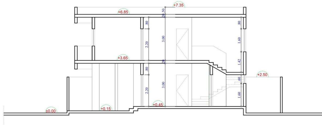
COUPE TRANSVERSALE
